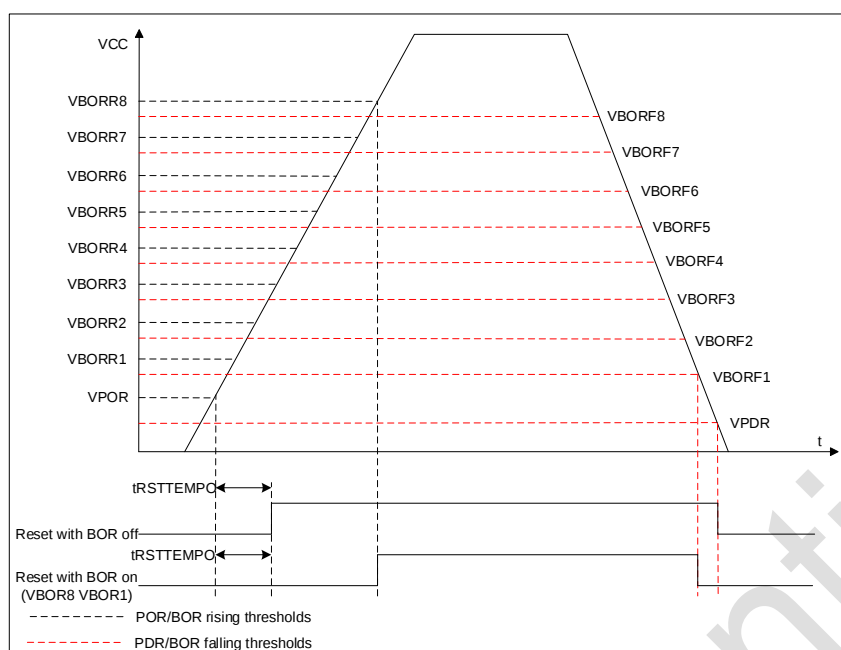
图 2-3 POR/PDR/BOR 阈值
