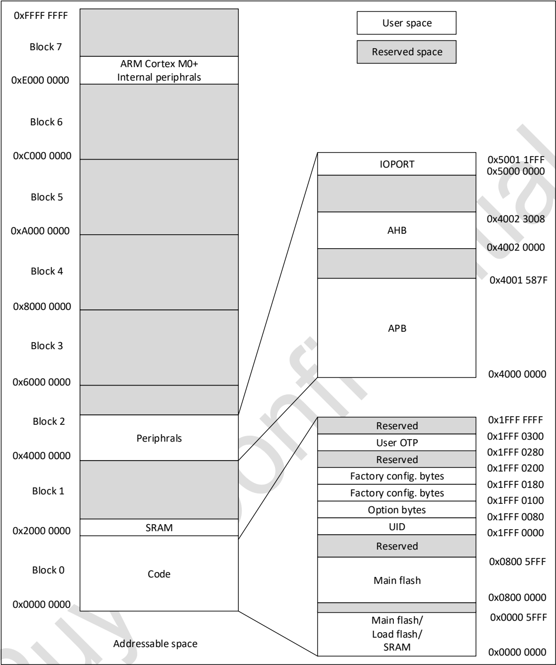
图 4-1 存储器映射
