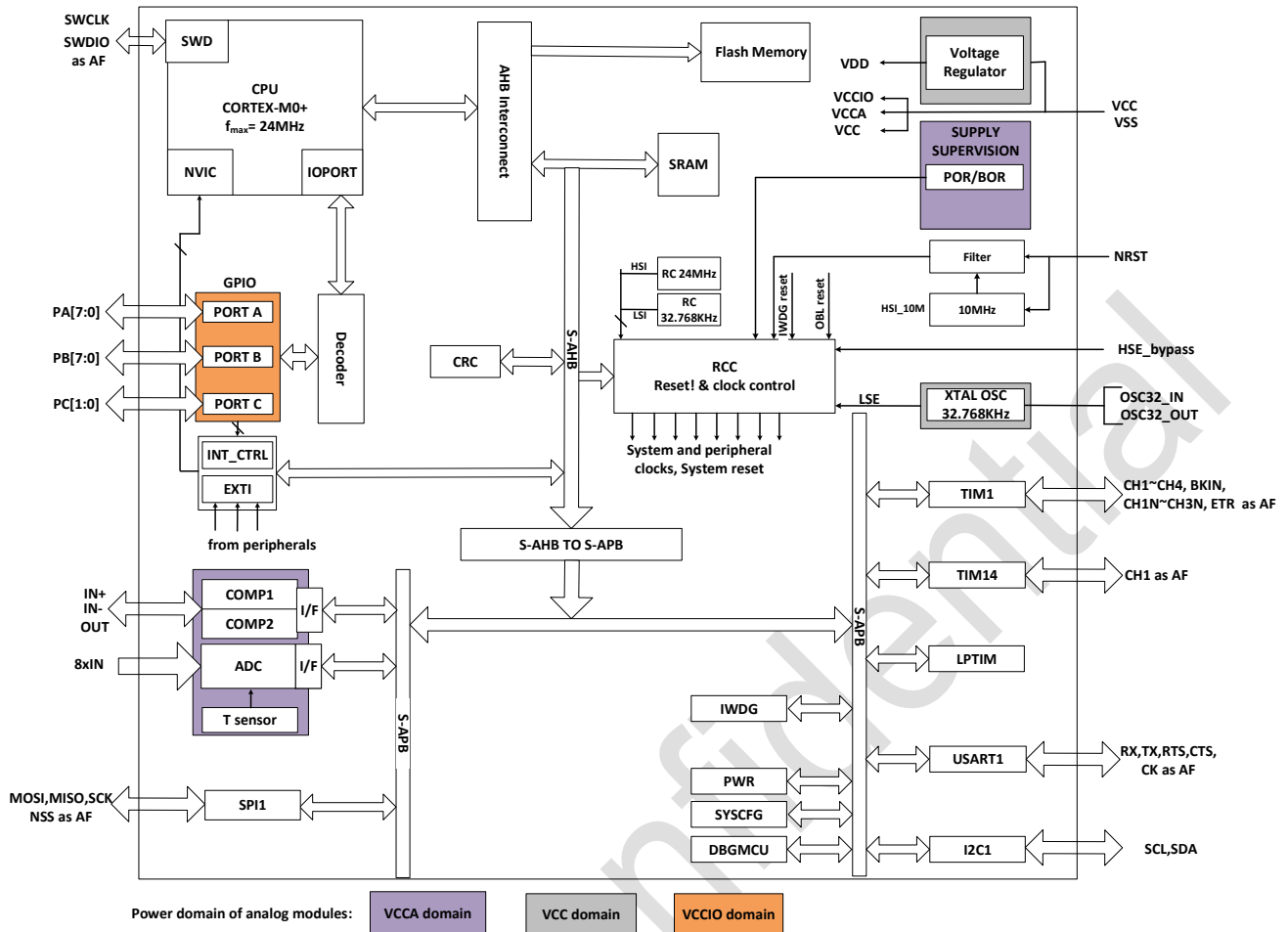
图 1-1 功能模块
